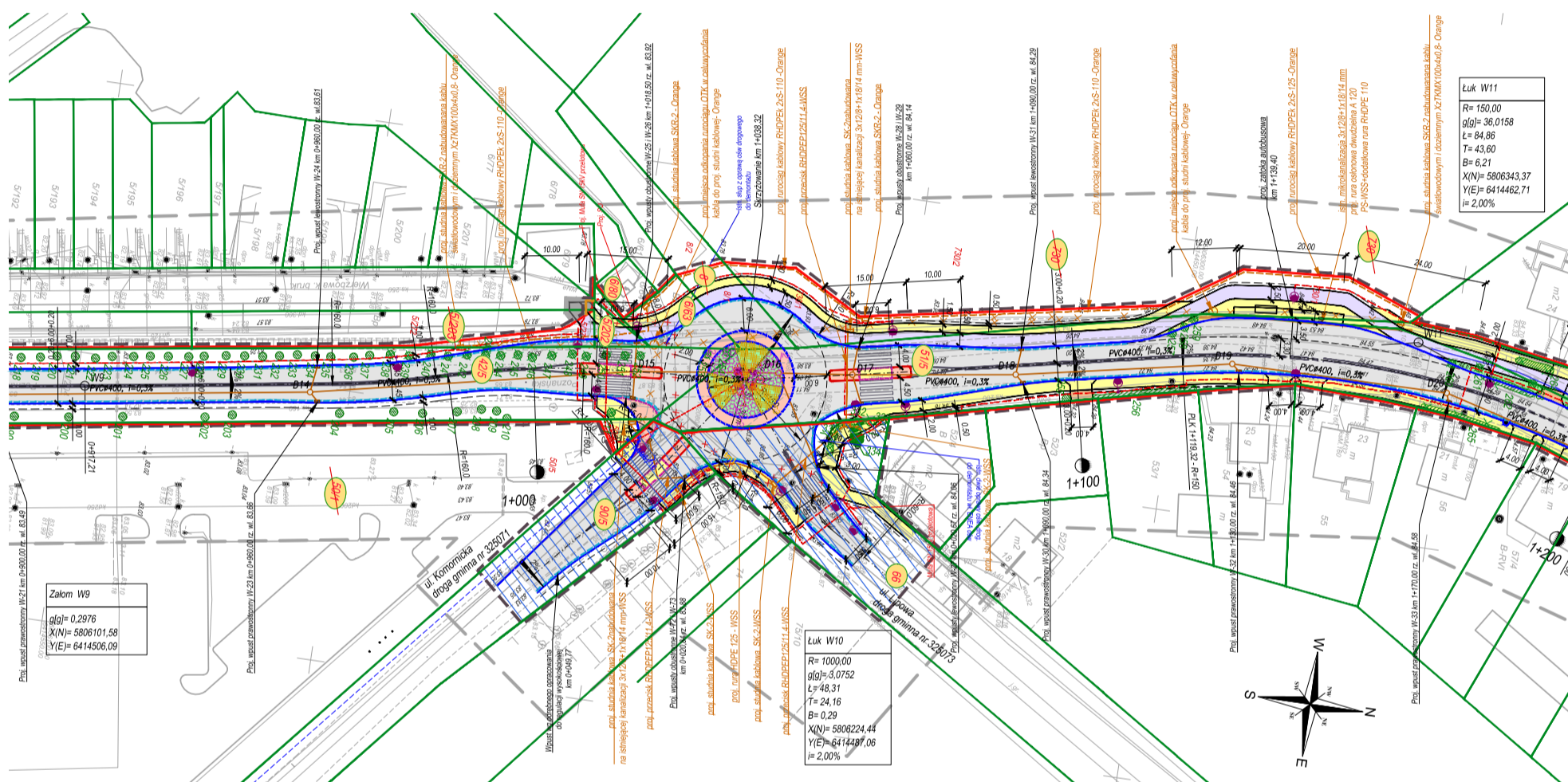
Fragment projektu ul. Poznańskiej w Dąbrówce z rondem przy ul. Komornickiej.
